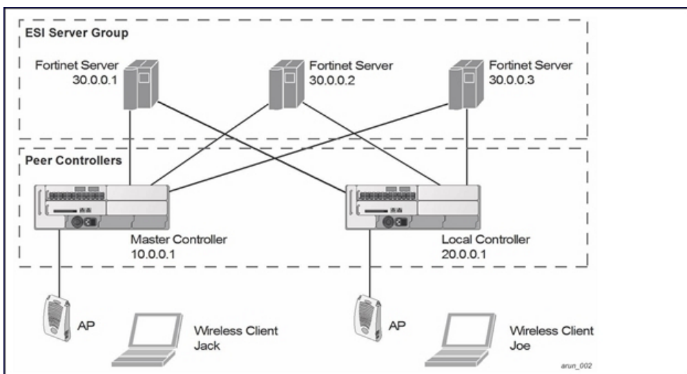
Figure 238 ESI Peer Controllers
